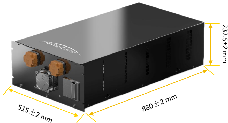
图 1 电池箱结构示意图
